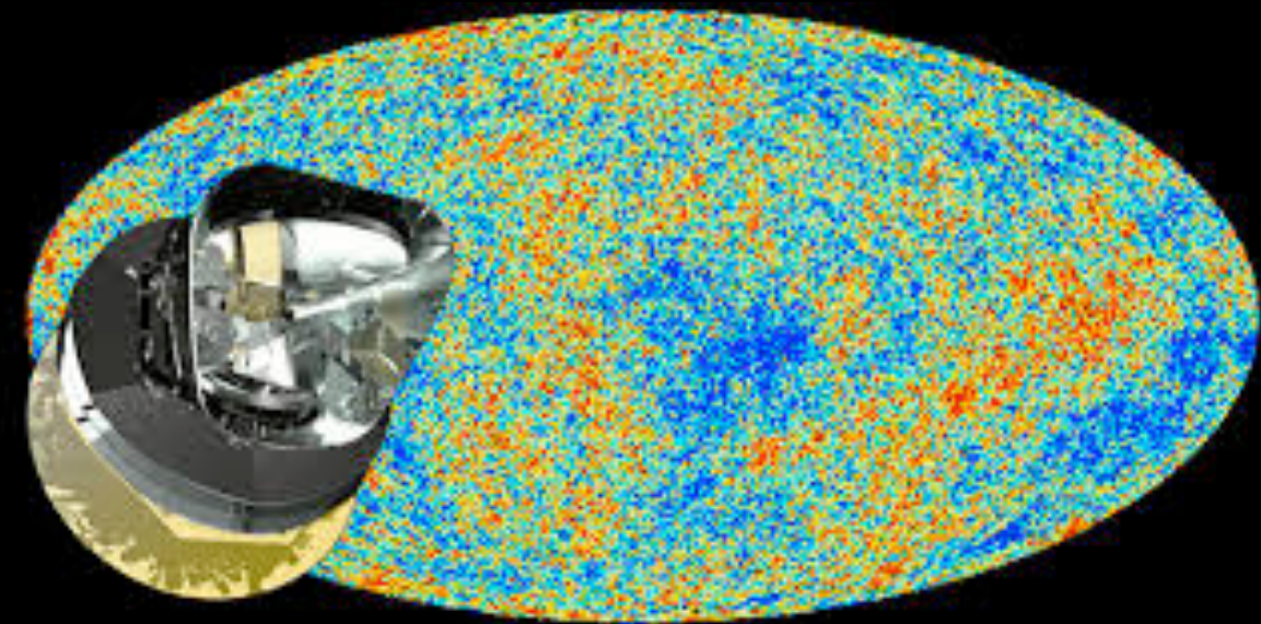
Planck
