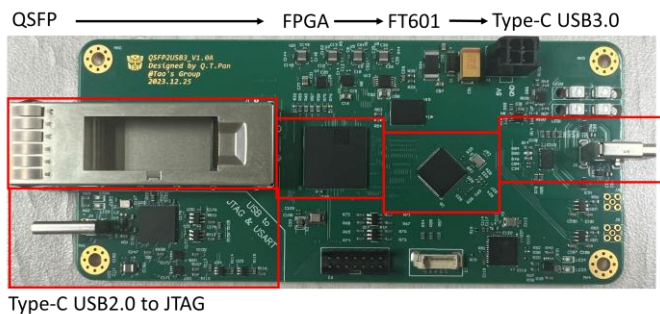
Fig. 2 PCB
