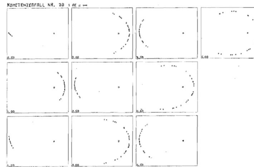
Abb. 1: Computersimulation einer Meteorstromentstehung aus dem Zerfall eines Kometenkerns. Die mit unterschiedlichen Geschwindigkeiten aus dem Kern austretenden Teilchen verteilen sich über die Bahn des Ursprungskometen. Die gezeigten Einzelstadien stellen die Teilchenpositionen in Abständen einer halben Umlaufzeit des Kometen dar (Zahlenangaben links unten in jedem Küstchen).
