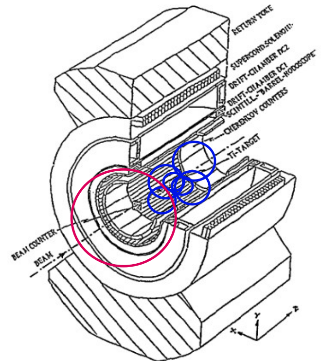
SINDRUM II (PSI)
