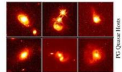
(f) Quasar
