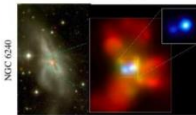
(d) Coalescence/(U)LIRG
