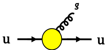
u-quark (Chromo)EDM
