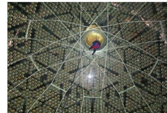
SNO+
