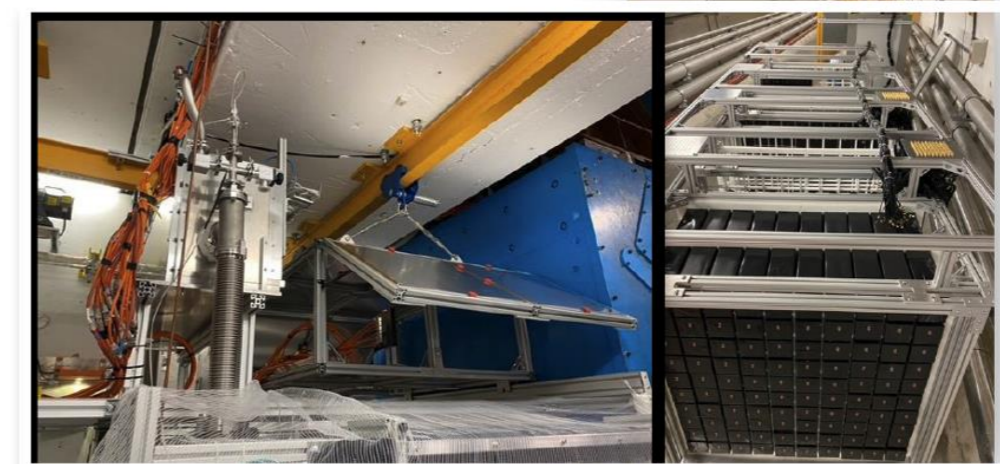
MoEDAL-MAPP
